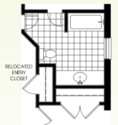
ALT. ENSUITE BATH
